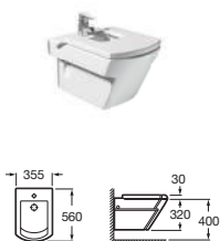
Подвесное биде
